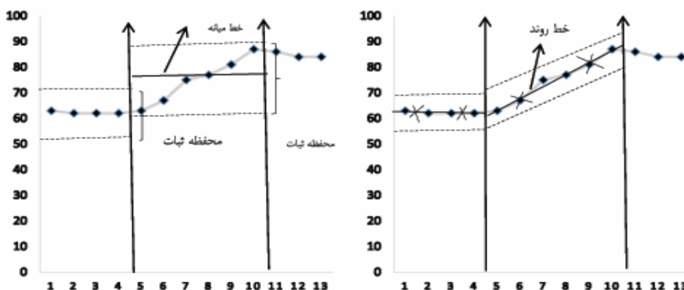
نمودار ۵. خط میان و خط روند و محفظه ثبات شرکت‌کننده سوم در زمینه مهارت‌های اجتماعی
