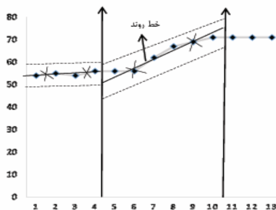
نمودار ۳. خط میانۀ و خط روند و محفظه ثبات شرکت‌کننده دوم در زمینه مهارت‌های اجتماعی
