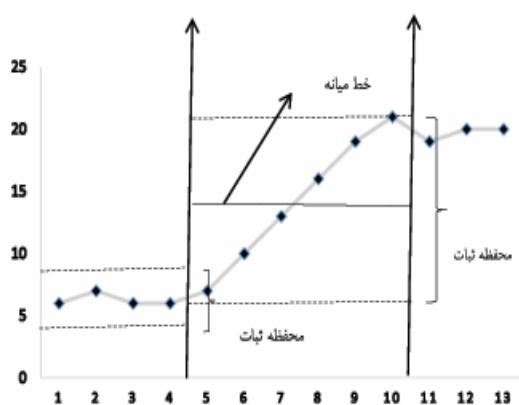
نمودار ۴. خط میانۀ و خط روند و محفظه ثبات شرکت‌کننده دوم در زمینه دانش جنسی
