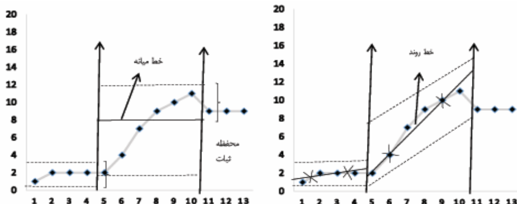
نمودار ۶. خط میانه و خط روند و محفظه ثبات شرکت‌کننده سوم در زمینه دانش جنسی
