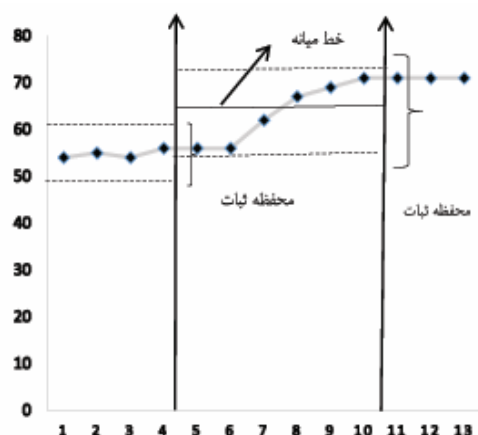
نمودار ۳. خط میانۀ و خط روند و محفظه ثبات شرکت‌کننده دوم در زمینه مهارت‌های اجتماعی
