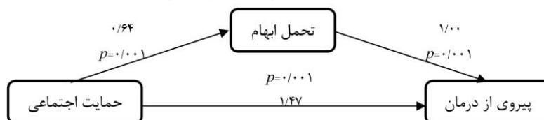
شکل ۲. مدل نهایی ضرایب استاندارد برآورد شده
