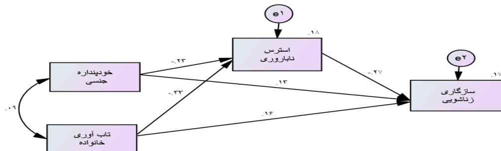
نمودار ۲. ضرایب استاندارد مسیر الگوی پیشنهادی آزمون شده
